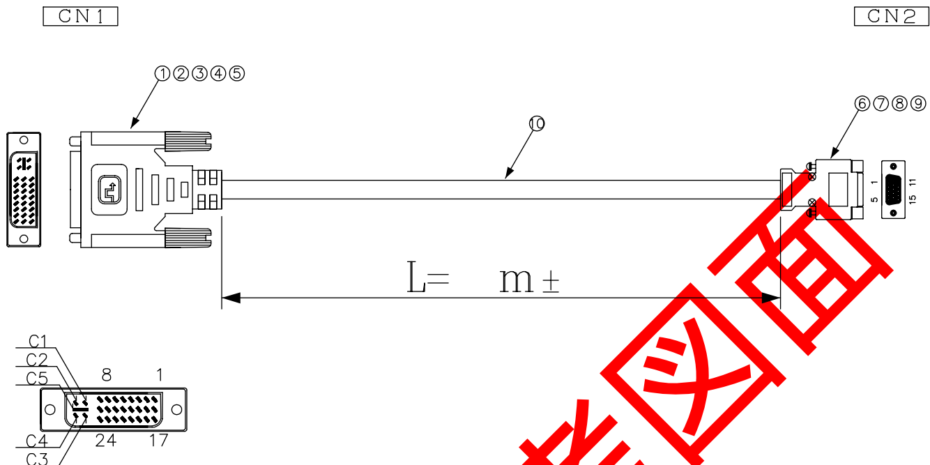
図1: かん合面から見た図
