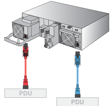
【冗長化電源ユニット接続例】
