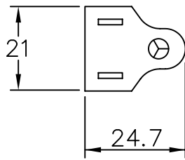
平型2P+アースピン (NEMA 5-15P)
